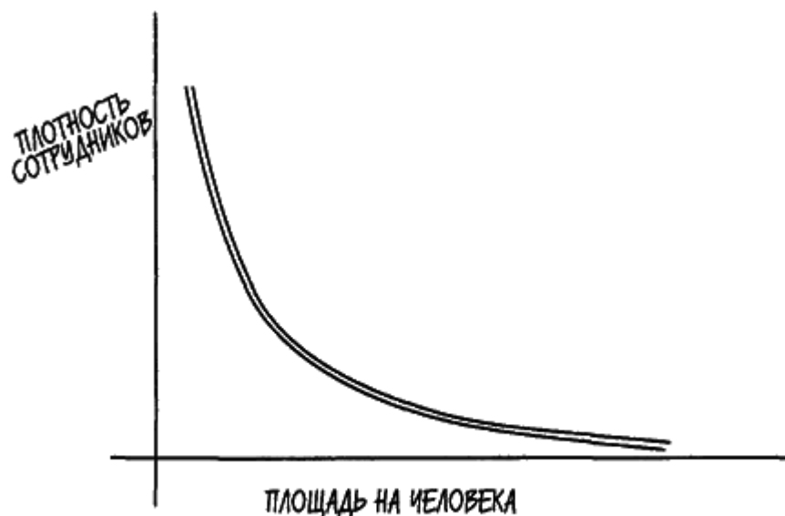
Рис. 9.2. Эффект Демарко-Листера
